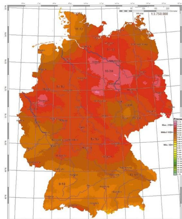
Fig. 3a e 3b Anomalia crescente nel soleggiamento e della radiazione globale in Germania - Servizio meteorologico tedesco
